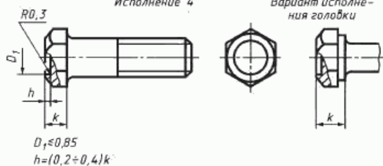
Исполнение 4
